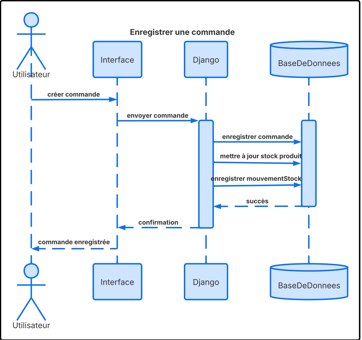
Sequence diagram - Enregistrer une commande
