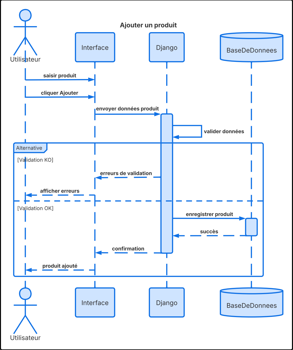
Sequence diagram - Ajouter un produit
